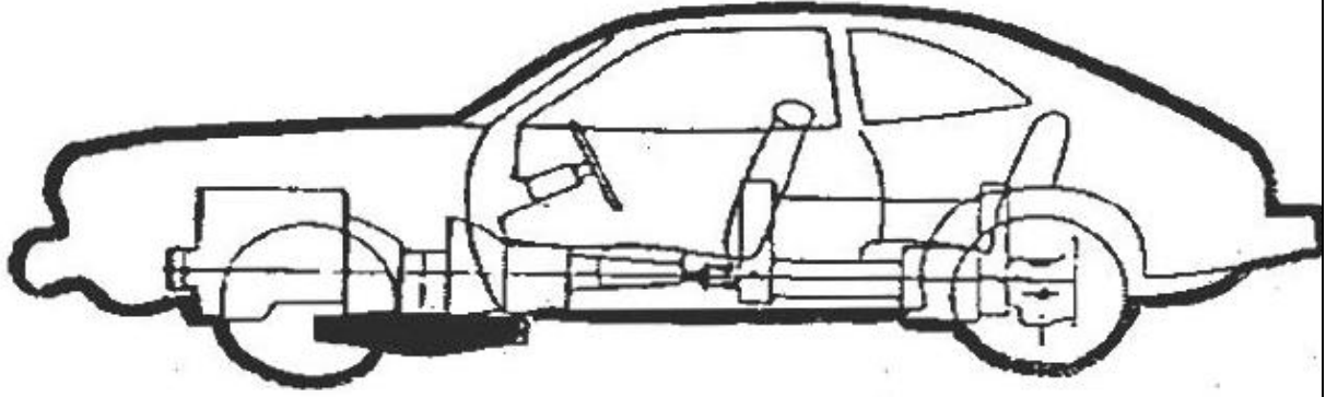
Şek. 2. Pinto şasesinde Volan Enerji İdare Birimi (FEMP) nin konumu.
