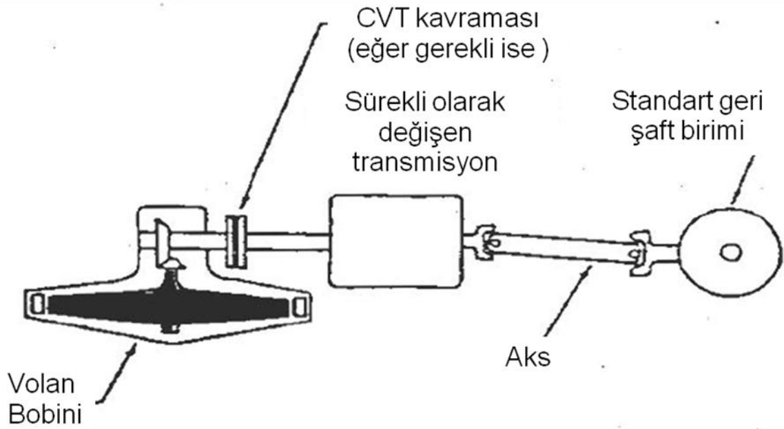
Şek. 1. Volan İletme Komuta Sisteminin temel görünümü.
